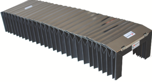
Paslanmaz kapaklı kızak köruk (Isı ve toza dayanıklı kumaştan üretilmiştir üstüne konulan paslanmazla dayanımı artırılmıştır)
