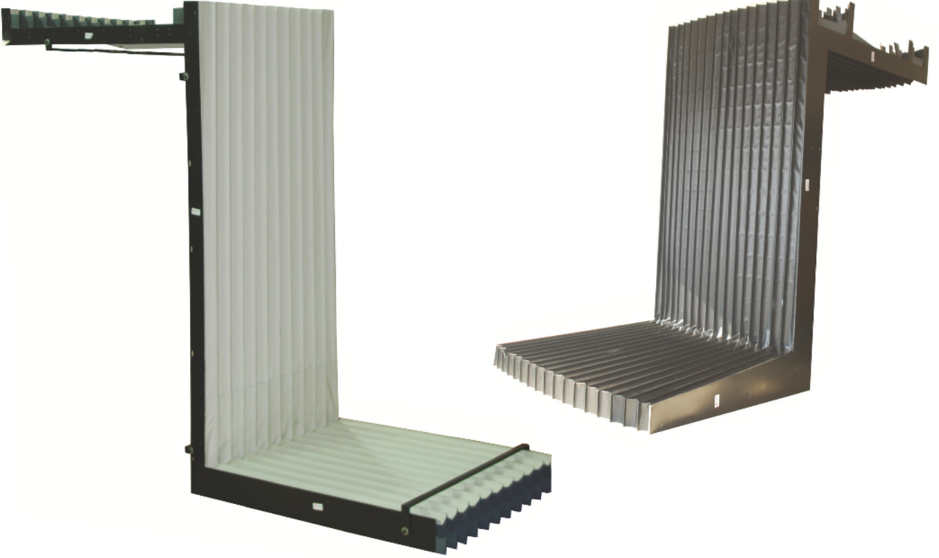
CNC Z körüğü (Yağ ve suya dayanıklı kumaştan üretilmiştir)
